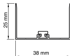
Profilo d'incontro/compensatore
