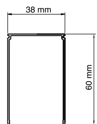
Guida superiore
