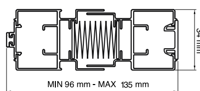
Profili portarete
