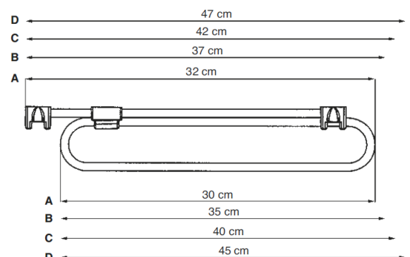
ART. 753 ESTRAIBILI PER ARMADIO
