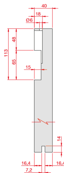
SEZIONE B-B
